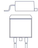
TO-263AB FG
